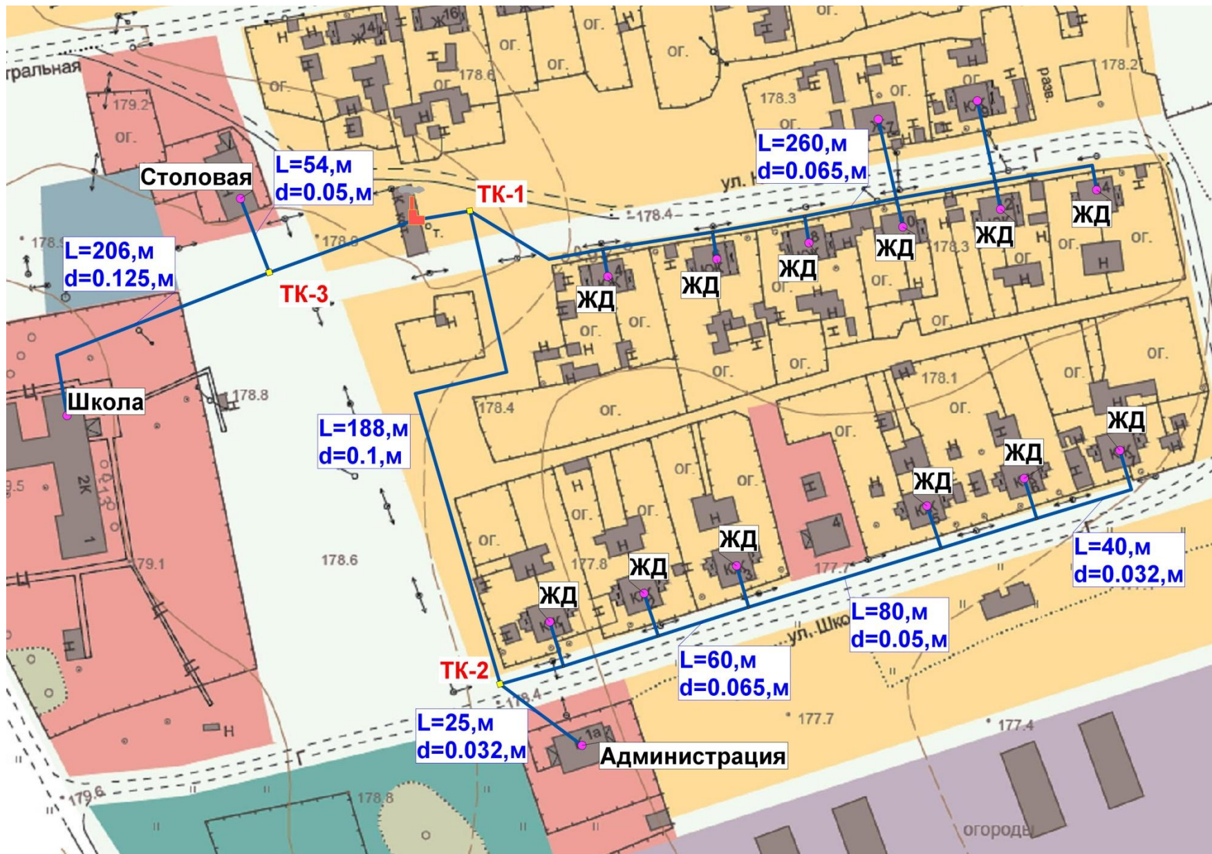
Рис.2.2 – Схема теплоснабжения котельной «Школа»
